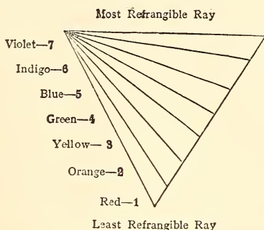
Fig. 33 : PRISMATIC SPECTRUM
